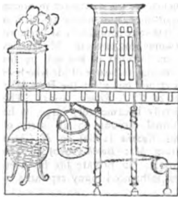
FIG. 1.—Hero's Apparatus, 130 B.C.
