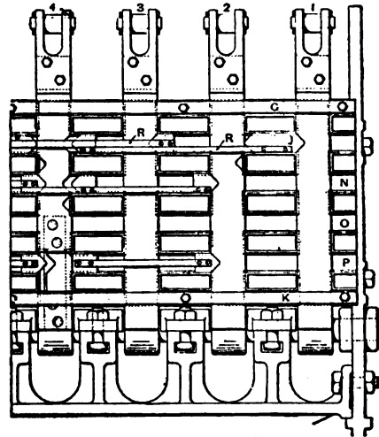
FIG. 7.—Interlocking Frame.
